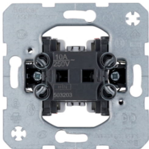
Tlačítko 2-pólové, řazení 1/0+1/0
